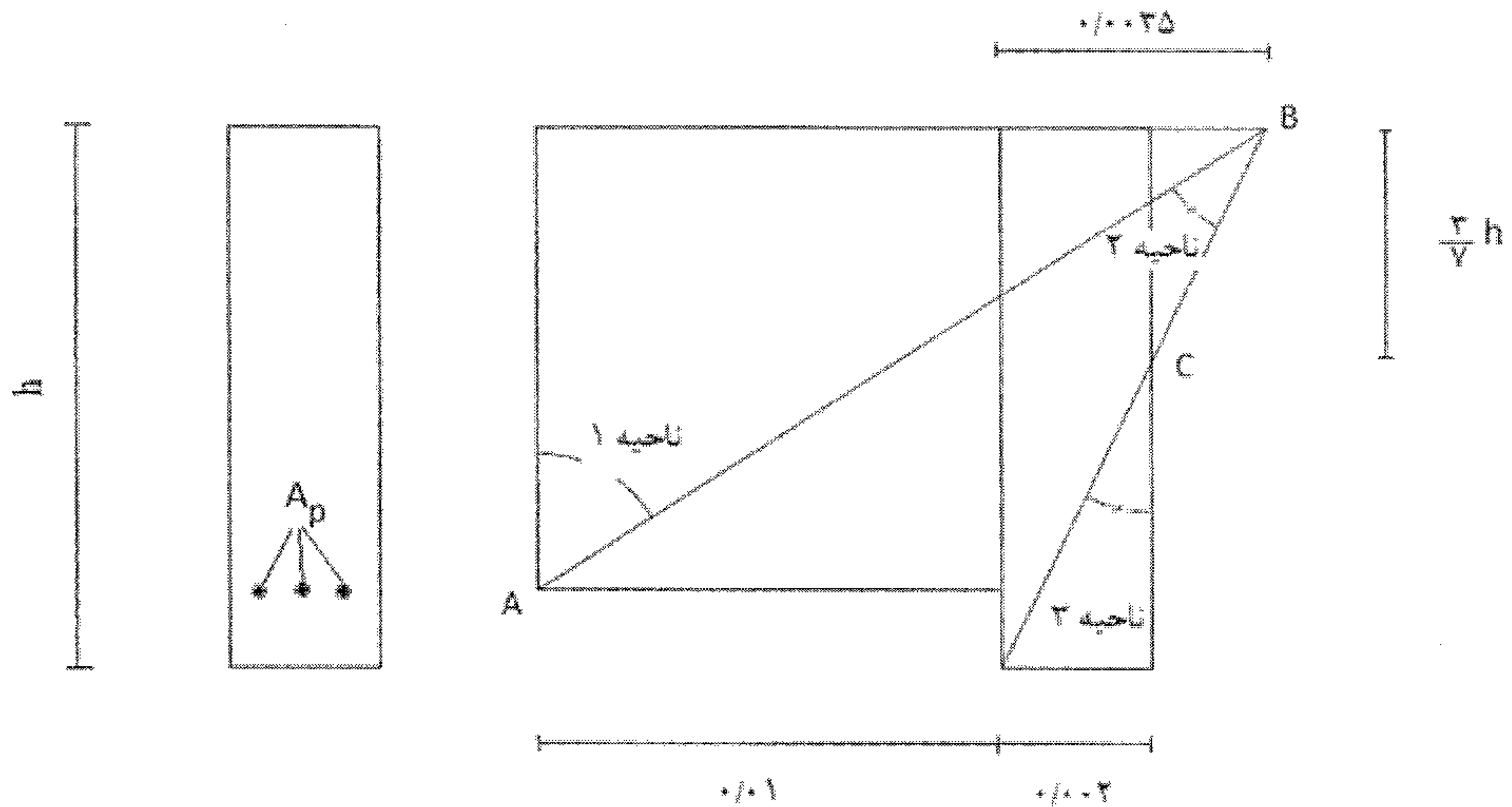
شکل ۹-۲۴-۱ نمودار تغییرشکل در حالت حدی نهایی
